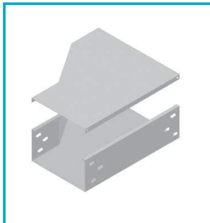
Tăng, giảm máng cáp Reducer cable trunking
